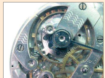
Detalle ampliado del volante en su posición
