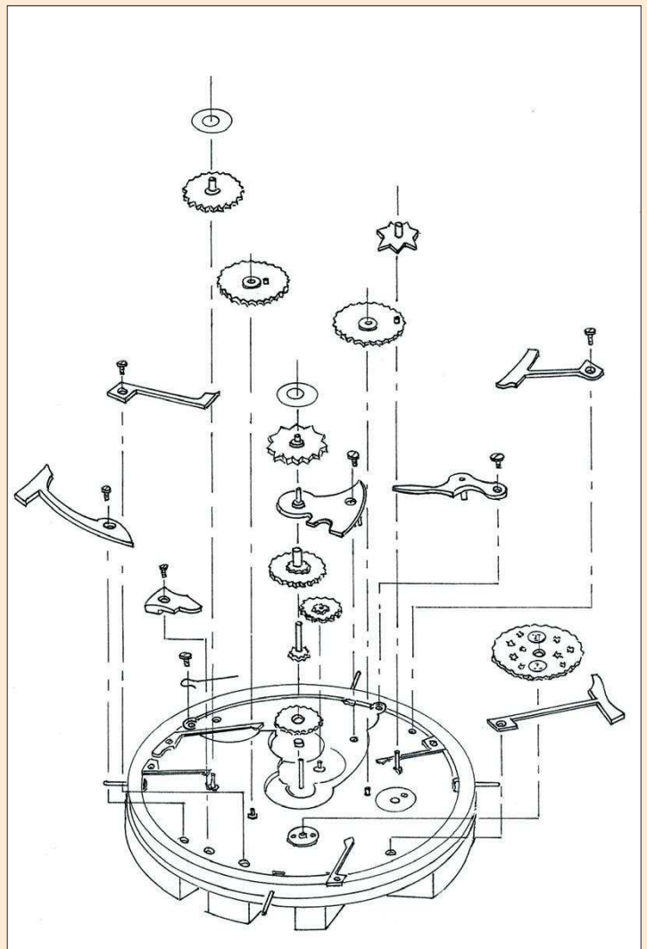
Despiece de la máquina donde podemos observar la posición de la palanca reparada
